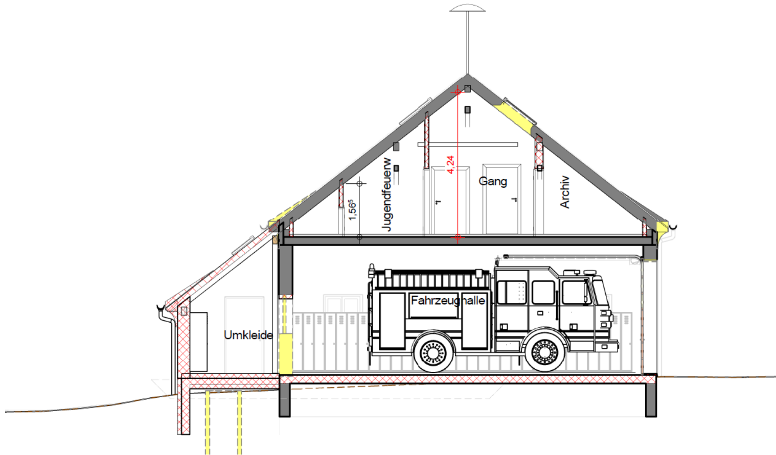
Schnitt C-C
