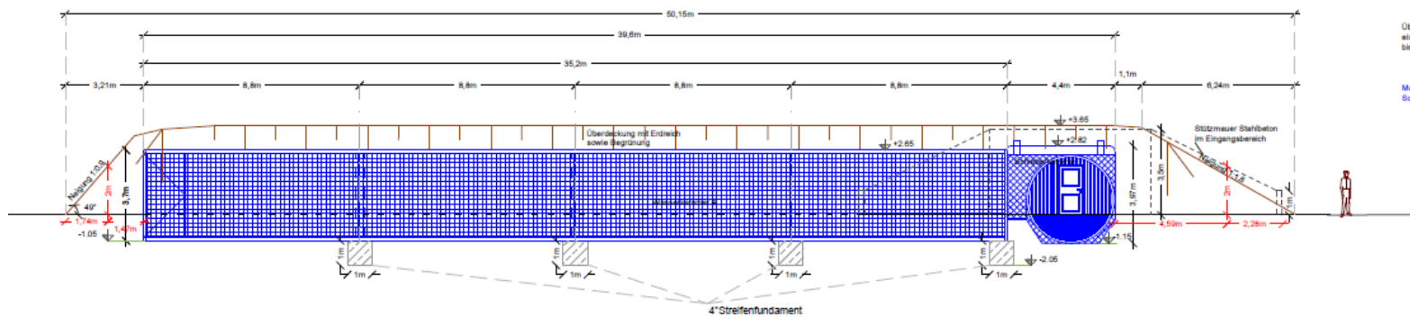
Längsschnitt (Bereich Eingang/ Westen) M=1:100
