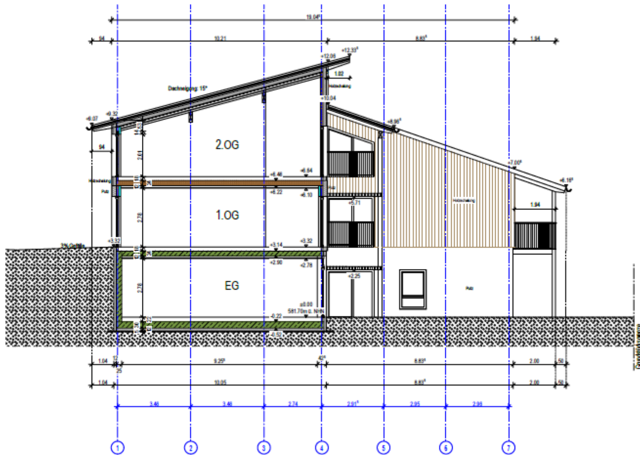
SCHNITT B-B
