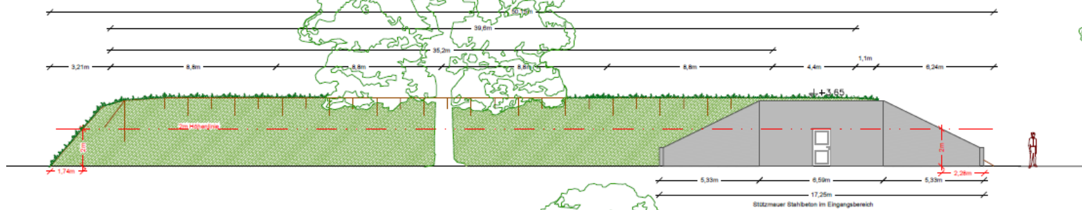
Ansicht Westen M=1:100
