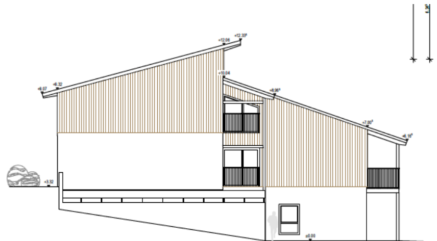
ANSICHT WEST
