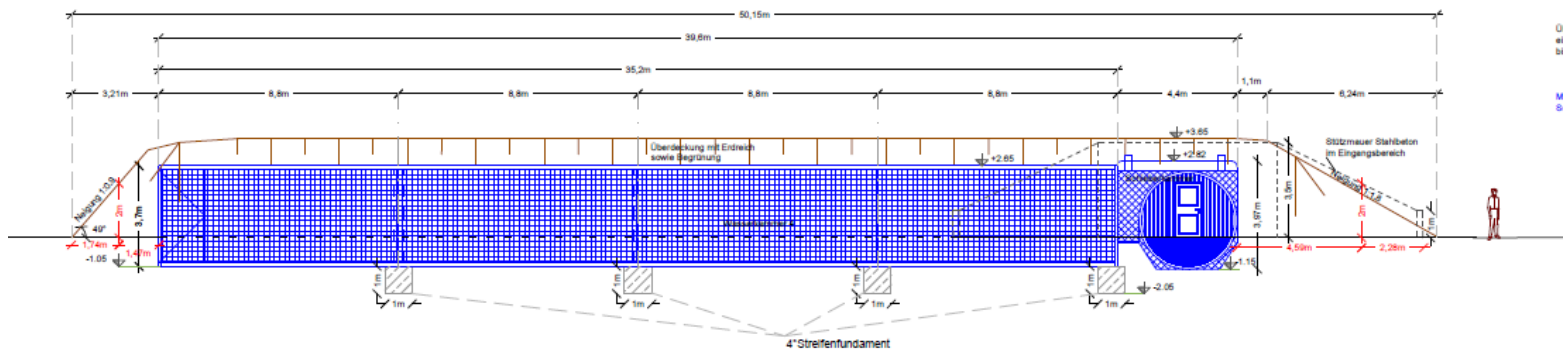
Längsschnitt (Bereich Eingang/ Westen)
